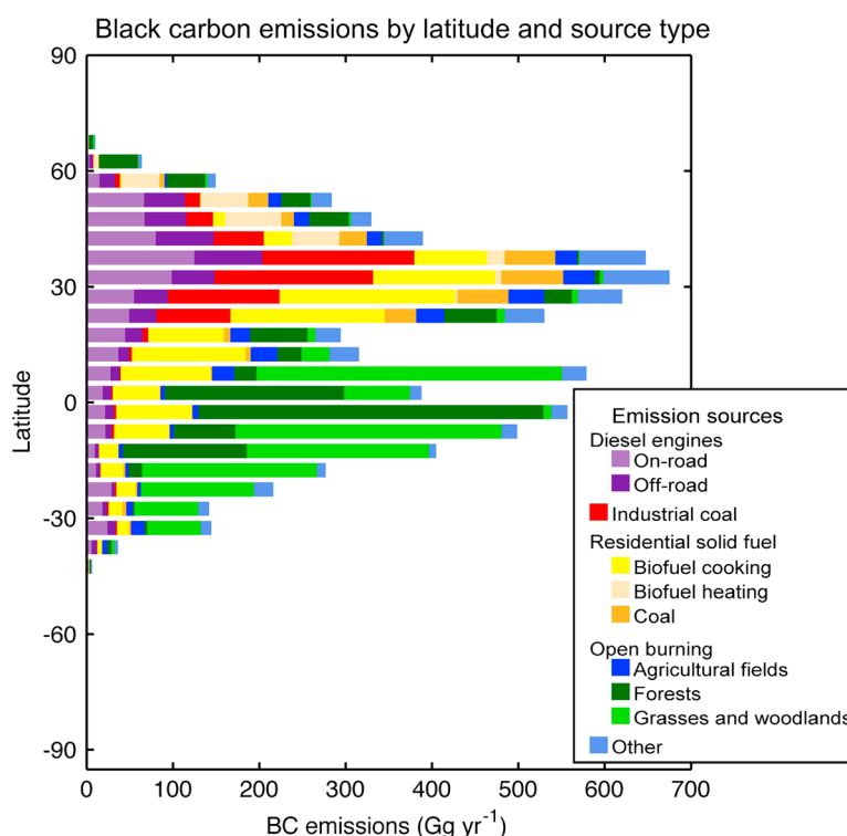
Figure 11. Latitude plot of the data shown in Figures 8 and 9 using 5° latitude bins.
